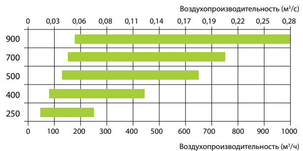
Типоразмеры установок Domekt CF
