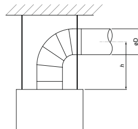
2. Свободно подвешенный к потолку диффузор h_{\text{мин}} > (3-5) D
