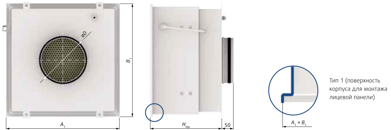
Рис. 7. Размеры CFC-G
