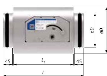
Рис. 3 Размеры NOTUS-RI-M0
