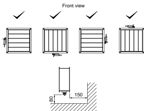
Рис. 2. Положение при монтаже
