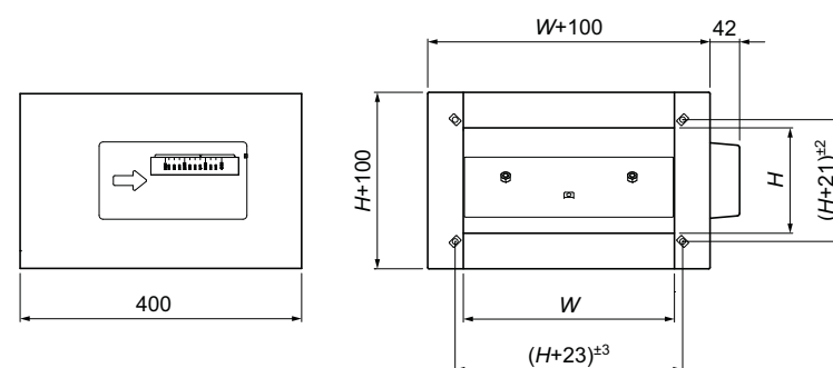
Рис. 2: Основные размеры RPK-SI
