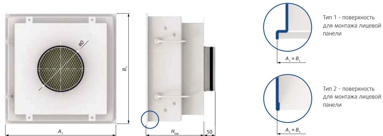
Рис 5. Размеры CFC-C. Примечание. см. табл. 3.
