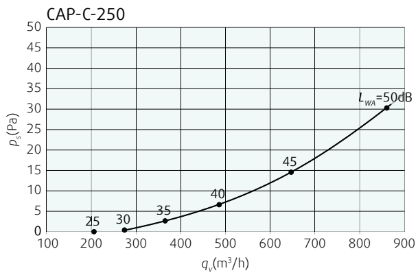
Диаграмма 5а. Перепад давления и уровень звуковой мощности
