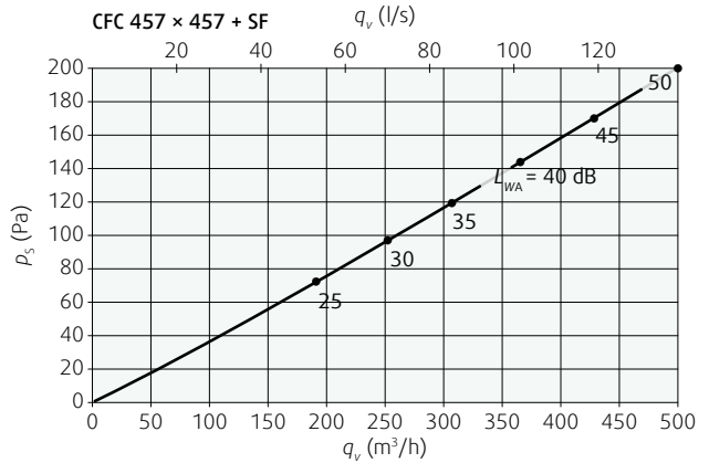
Диаграмма 6: Потери давления & A-взвешенный уровень звуковой мощности в зависимости от расхода воздуха; при измерении с лицевой панелью CFC-SF
