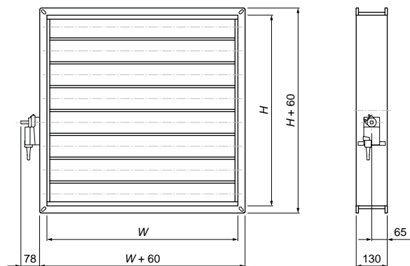
Рис. 1. TUNE-S, размеры
