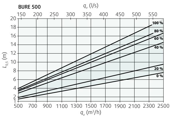
Диаграмма 4б: Дальность броска изотермической вертикальной струи при конечной скорости 0,5м/с. (Все типы диффузоров BURE).
