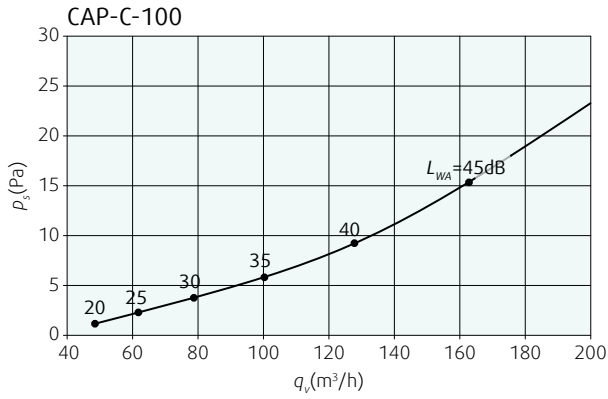
Диаграмма 1а. Перепад давления и уровень звуковой мощности
