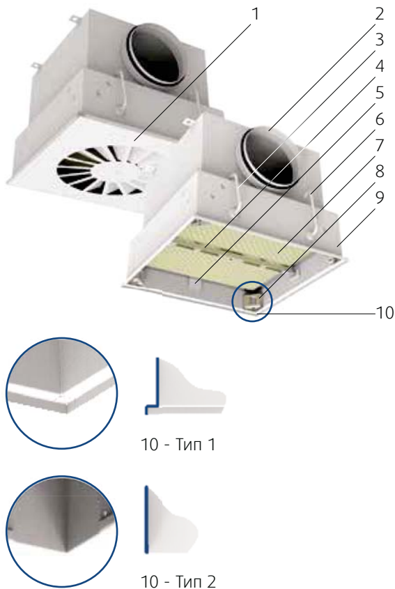
Рис. 1. Конструкция CFC.
