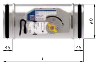
Рис. 2 Размеры NOTUS-R-M1
