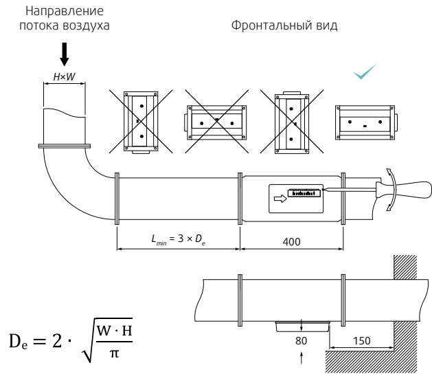
Рис. 3: Варианты монтажа RPK-S and RPK-SI
