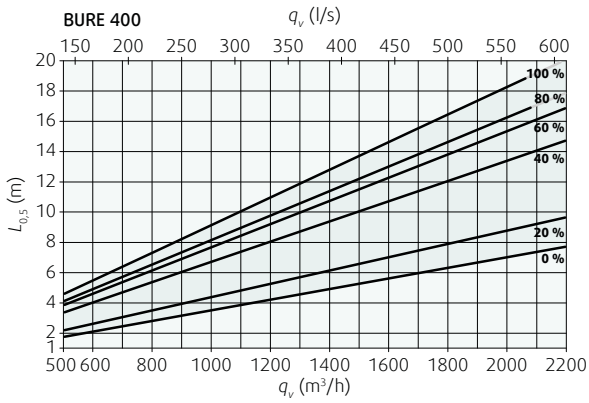
Диаграмма 3б: Дальность броска изотермической вертикальной струи при конечной скорости 0,5м/с. (Все типы диффузоров BURE).
