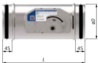
Рис. 1 Размеры NOTUS-R-M0
