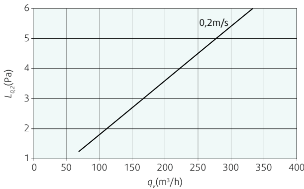
Диаграмма 2б. Длина струи при изотермическом распределении воздуха на 4 стороны. Конечная скорость 0,2 м/с.
