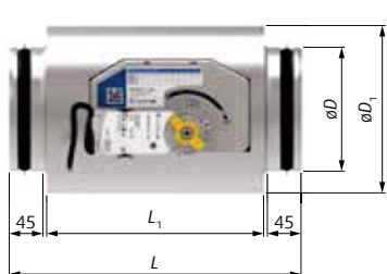
Рис. 3 Размеры NOTUS-RI-M1
